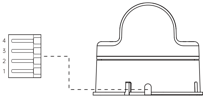
4PIN 串口图及出线管脚序号图
