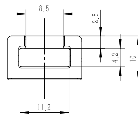
导轨截面尺寸
